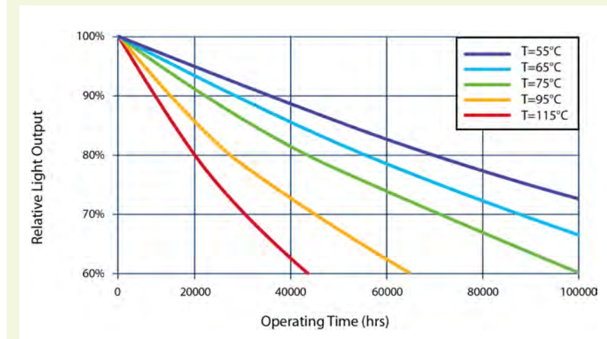
-Figuur 2- Een goede koeling van leds is essentieel, want de lichtopbrengst gaat sneller achteruit bij hogere temperaturen
